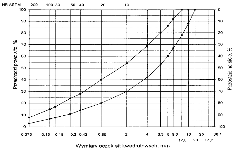
Rys. 9. Krzywe graniczne uziarnienia mieszanki mineralnej BA od 0 do 12,8 mm do warstwy wiążącej, wyrównawczej i wzmacniającej nawierzchni drogi o obciążeniu ruchem KR1 lub KR2
